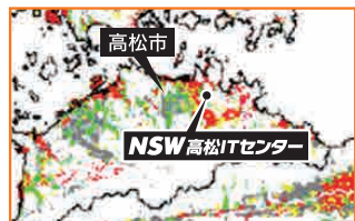
基本ケース/液状化可能性【近畿・四国】
