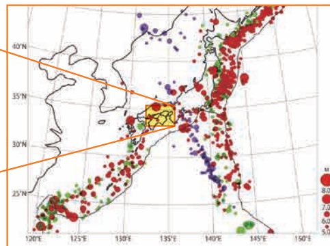
日本列島とその周辺の地震活動 (2000年～2009年 M5以上) ※2
