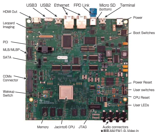
Jacinto6 CPU EVM
